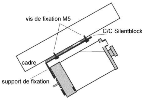
Vue latérale de fixation
