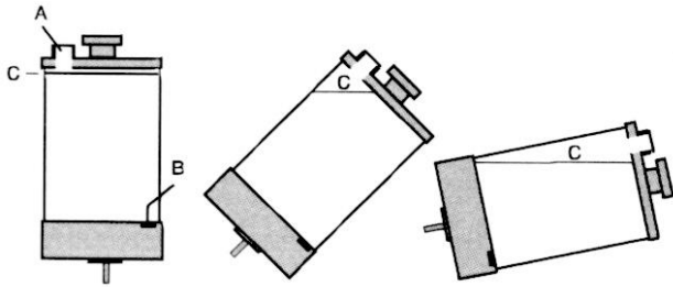
Vue latérale de montage
